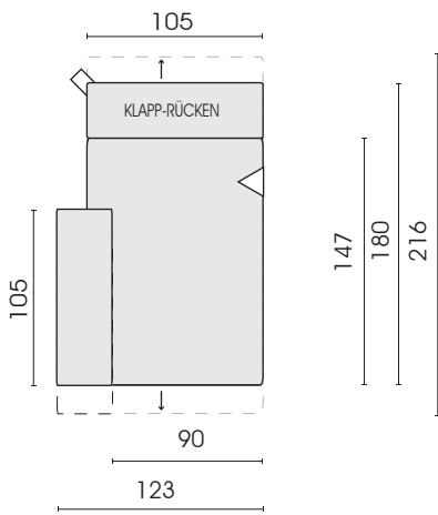
Ecksofa 2,5-Sitz, links mit motorischer Sitzverstellung 54M
