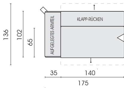
Sofa 2,5-Sitz AT aufgelegt, links mit motorischer Sitzverstellung 58M
