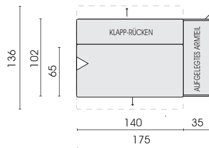
Sofa 2,5-Sitz AT aufgelegt, rechts mit motorischer Sitzverstellung 57M
