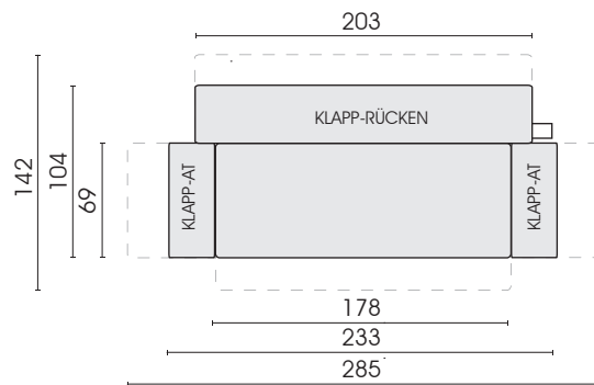
Abgeklappt Typ 300
