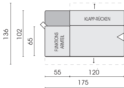
Sofa 2-Sitz Funktionsarmteil links mit motorischer Sitzverstellung 26M
