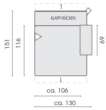
Funktionsliege, breit Armteil rechts mit motorischer Sitzverstellung 441F
