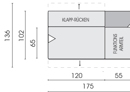
Sofa 2-Sitz Funktionsarmteil rechts mit motorischer Sitzverstellung 25M
